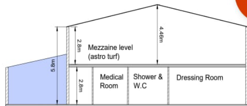
SECTION A-A Scale 1:100@A1
